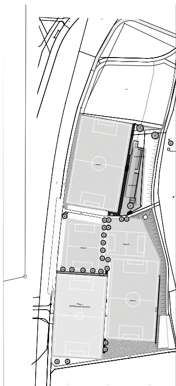
Situationsplan Bilg Kunstrasen Platz 3
